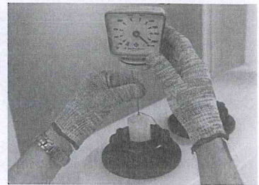
Etape 26- Laisser glisser le poids de la jauge mécanique dans le réservoir. Visser et serrer la jauge dans l'entretoise filetée.
