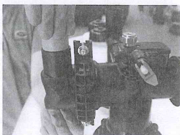
Etape 14- Emboîter le bouchon obturation aération (11) dans le coude d'aération (8).
