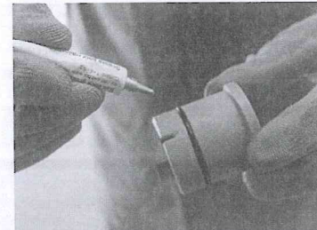
Etape 15- Mettre de la graisse 6 sur le joint du bouchon obturation aération 11 .
