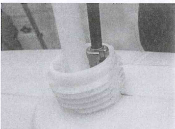
Etape 4- Etirer le tube télescopique (2) au maximum puis faire passer avec le tuyau de soutirage dans une bonde du réservoir.
